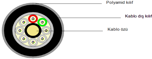
Resim 6: Polyamid kılıflı örnek kablo çizimi
