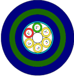
Resim 2: Yangına dayanıklı, zırhlı fiber optik kablo kesiti
