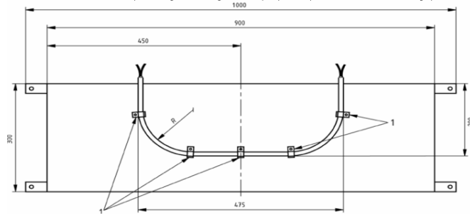
Resim 7: EN 50200 test düzeneği
