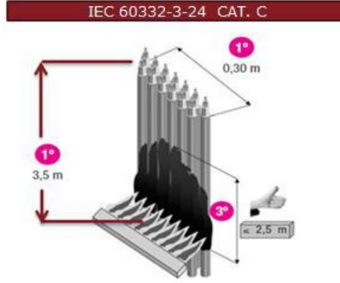
Resim 8: IEC 60332-3-24 (CAT. C) test düzeneği
