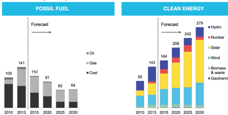
Kaynak : Bloomberg New Energy Finance, Michael Liebreich Tablo 1: Dünyada fosil yakıt ve temiz enerji üretim kapasitesi (GW)
