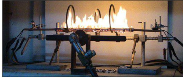
IEC 60331 test düzeneği
